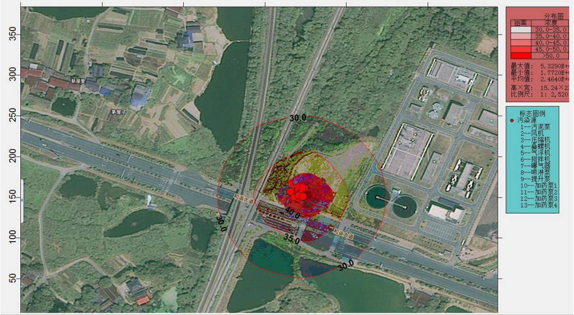
图4-3（a） 昼间噪声贡献值等声级线图
