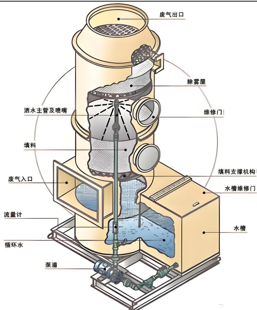
图 4-1 喷淋洗涤示意图
