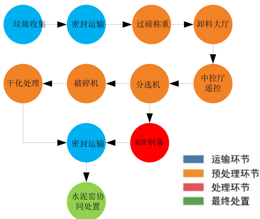
图 4-4 华新环境生活垃圾工艺流程
