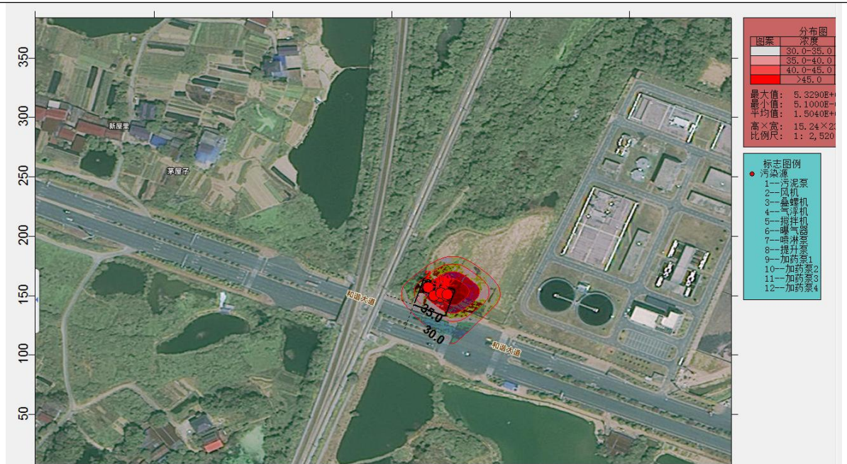
图4-3 (b) 夜间噪声贡献值等声级线图
