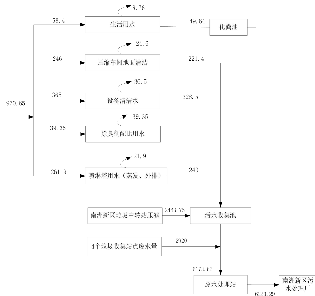
图 2-1 项目水平衡图 \text{m}^3/\text{a}
