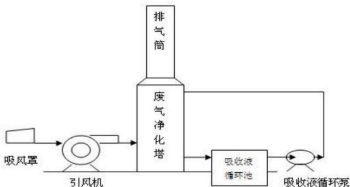
图 7.2-2 喷淋净化塔示意图
