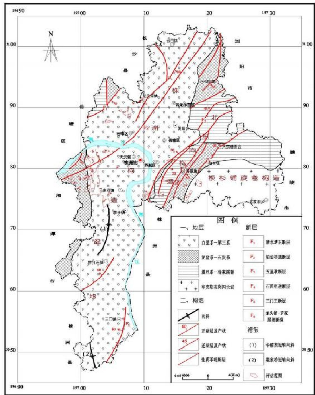
图 5.2-5 评价区地质构造体系图
