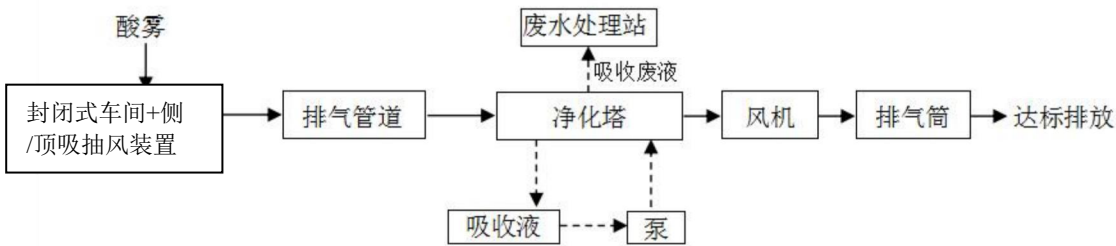
图 7.2-1 项目酸碱废气处理流程图
