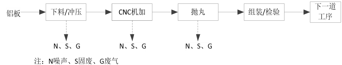
图 3.3-2 机加工工艺流程及产污节点
