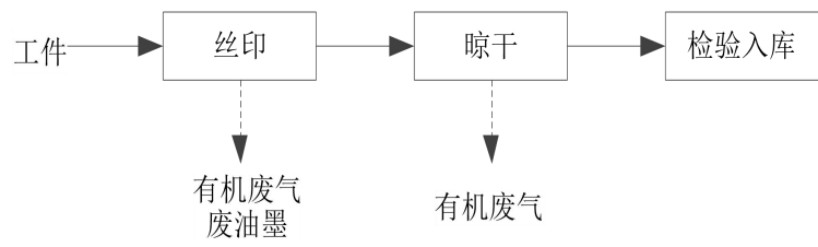
图 3.3-4 丝印线工艺流程及产污节点
