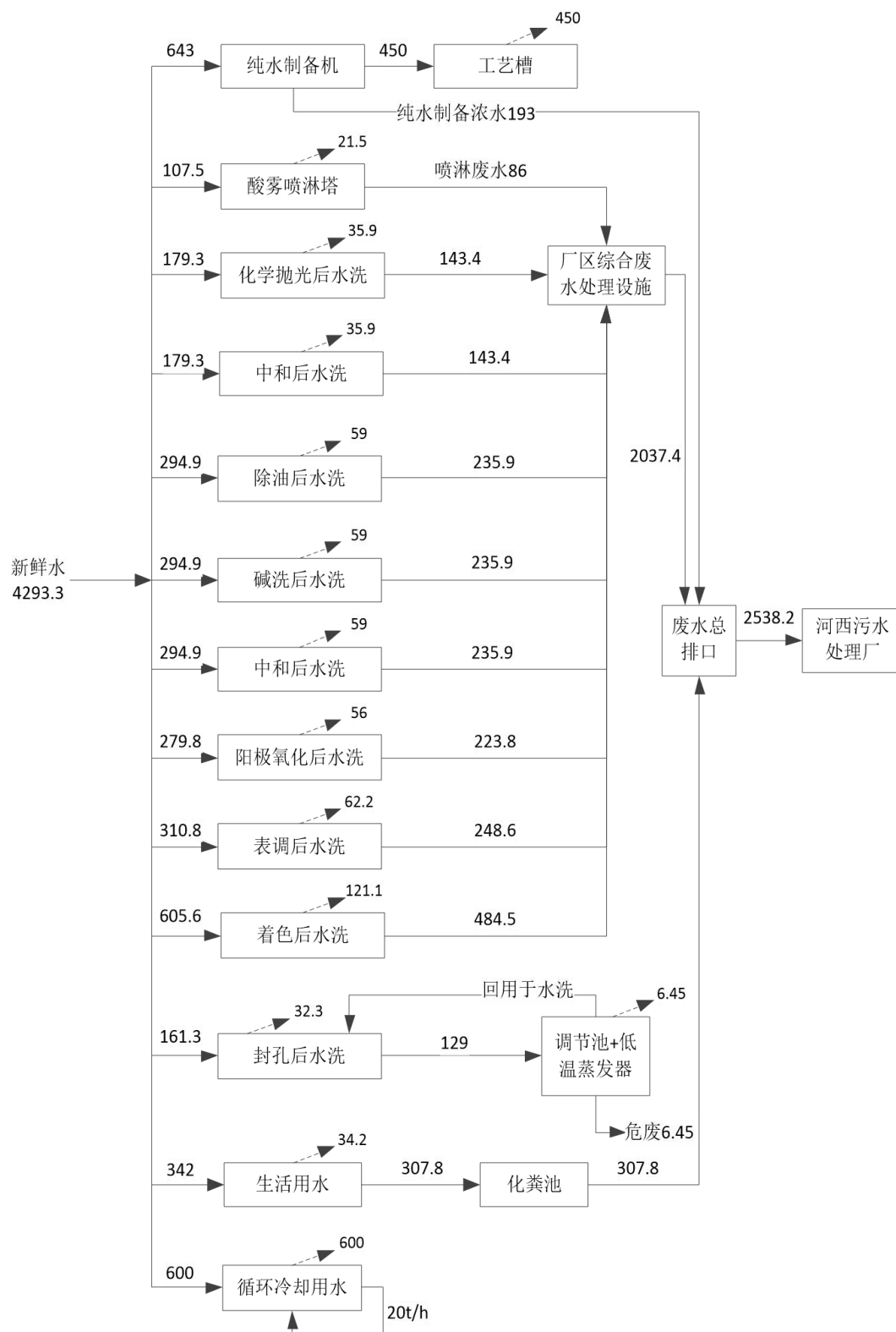
图 3.4-1 项目水平衡图
