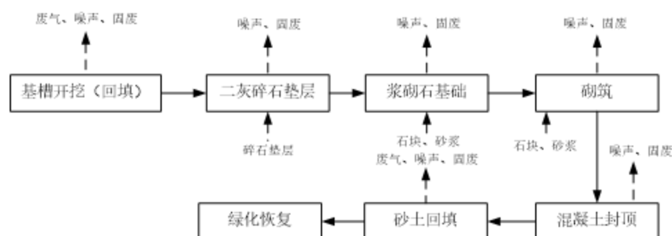
图1-3浆砌石挡墙施工工艺流程及产污节点
