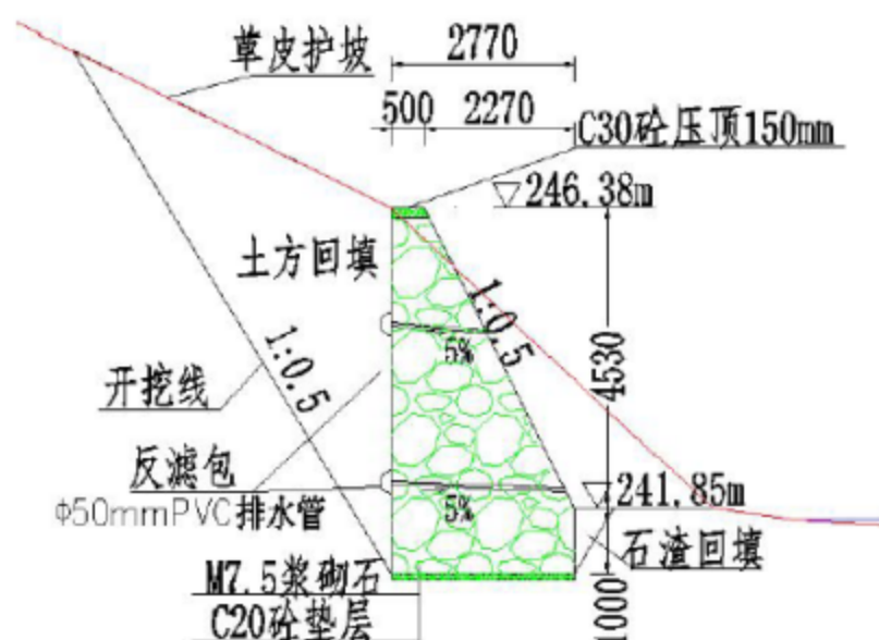
图 3-1 浆砌石挡墙断面
