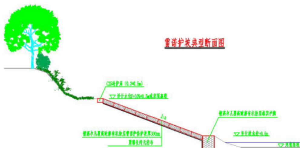
图 3-2 雷诺护坡典型断面图
