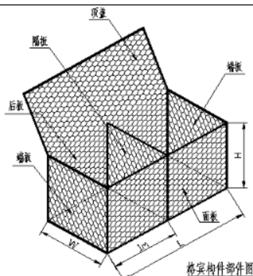
图 3-4 格宾构件部件图
