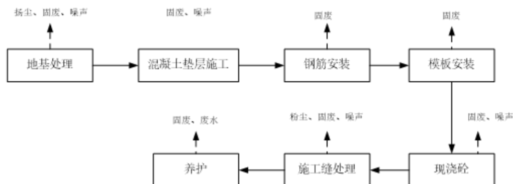
图1-4下河踏步施工工艺流程及产污节点
