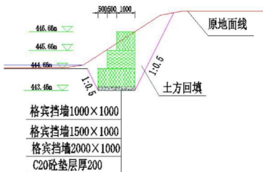
图 3-3 格宾挡墙断面示意图
