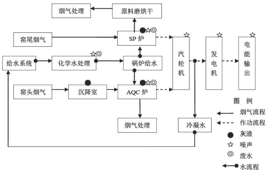
图 2.9-4 回转窑余热锅炉发电工艺流程
