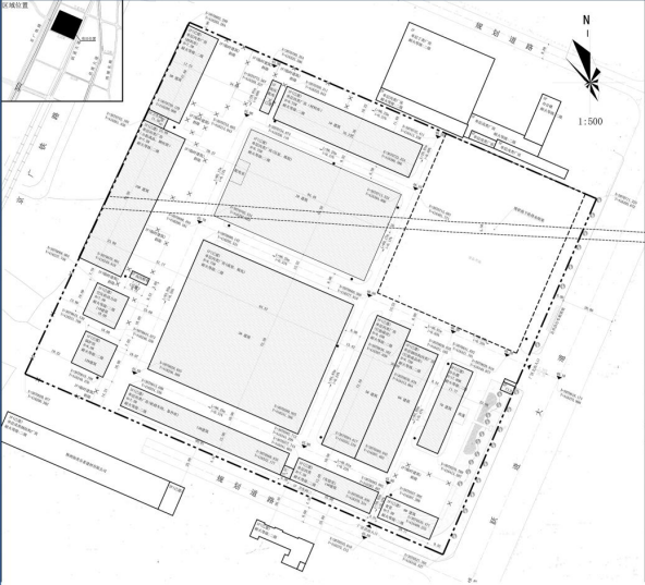
调整前总平面图 (上图根据已建建筑房产证绘制)
