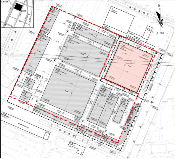
调整后总平面图
