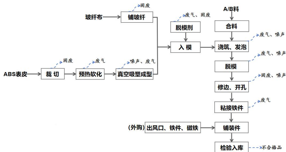
图 2-2 本项目仪表台、风道工艺流程及产污节点图
