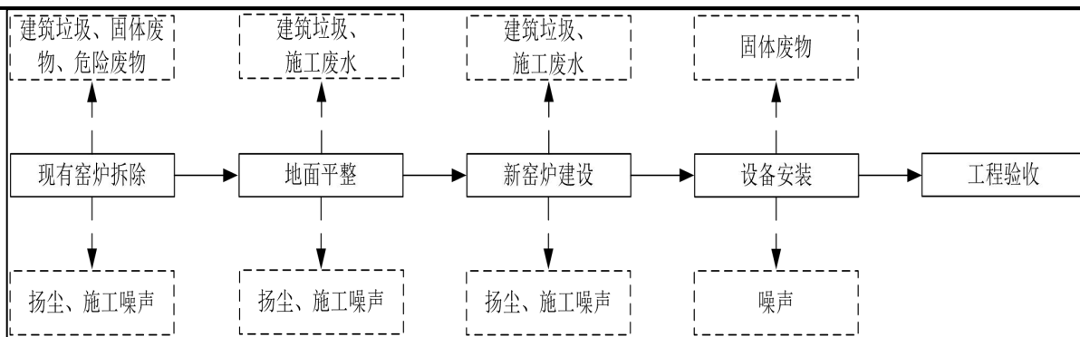
图 2-2 施工期生产工艺及产排污图
