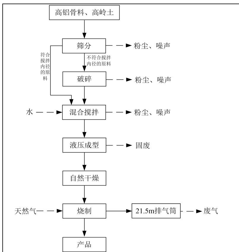
图2-3运行期生产工艺及产排污图
