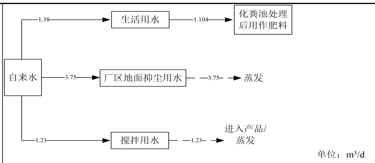
图4-1本项目全厂水平衡图
