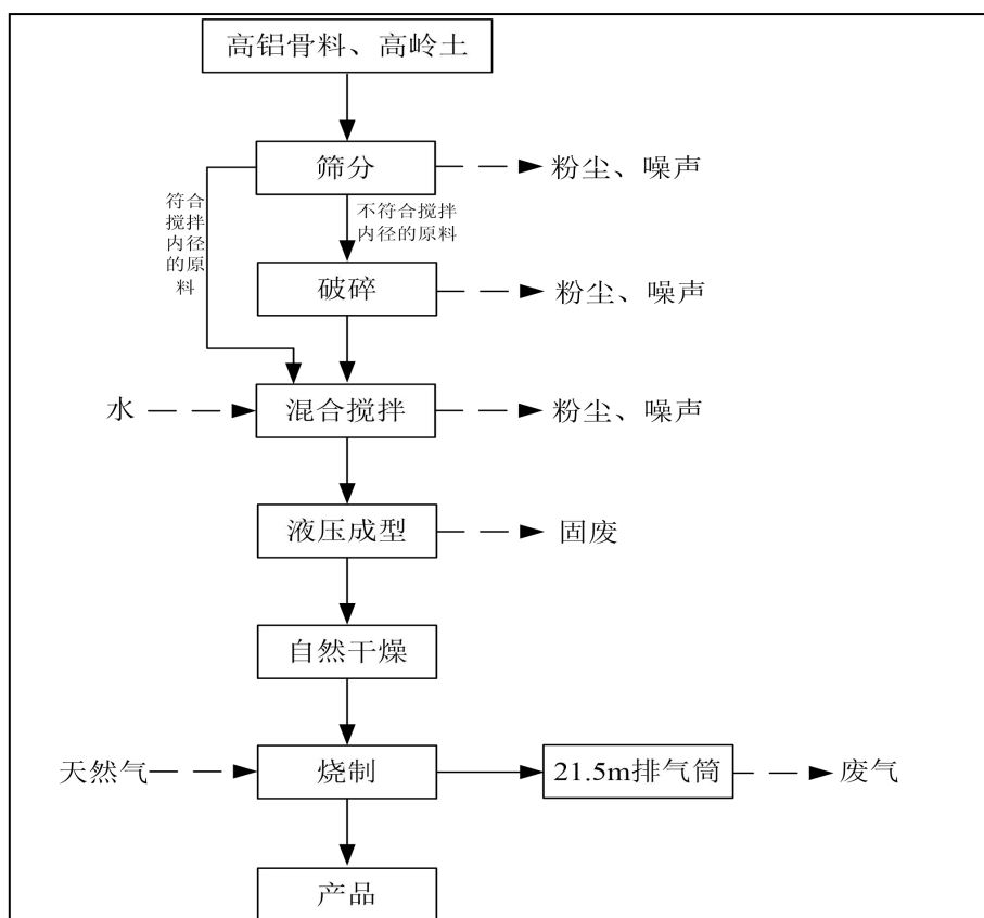
图2-3运行期生产工艺及产排污图
