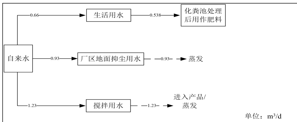
图2-1 本项目全厂水平衡图
