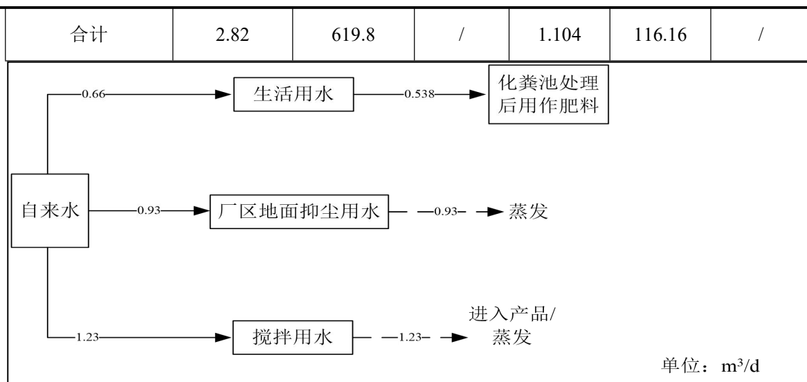
图4-1本项目全厂水平衡图
