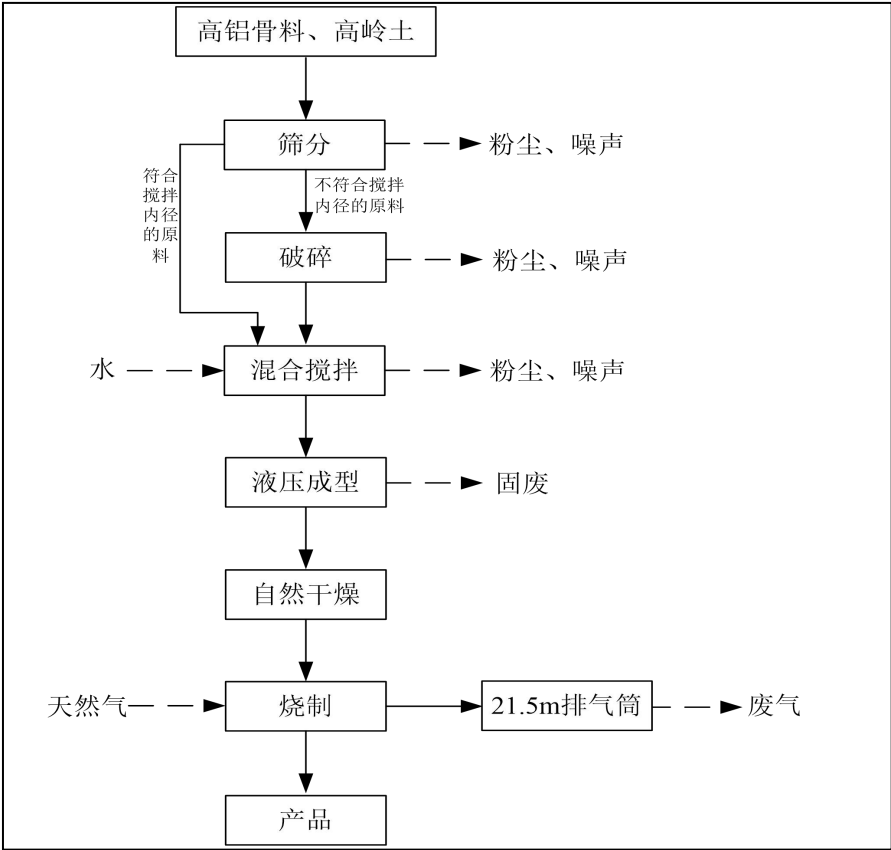
图2-3运行期生产工艺及产排污图
