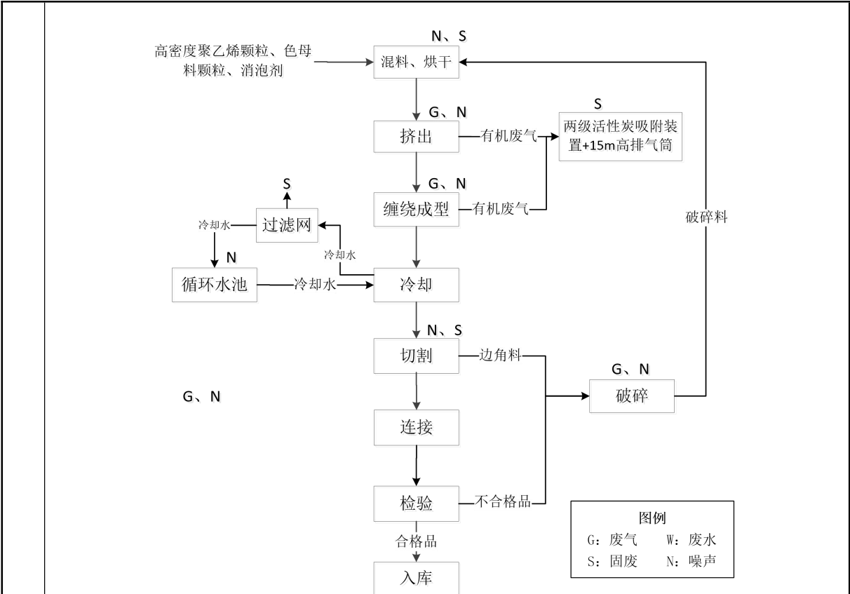
图 2-4 缠绕管生产工艺流程及产排污节点图
