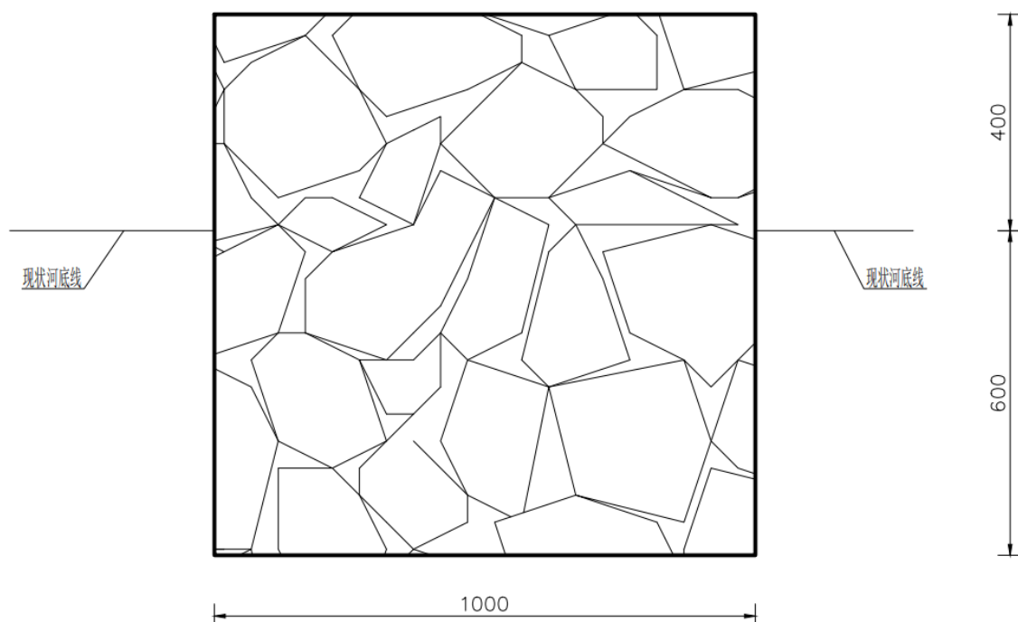
图 2-21 黄龙江水生植物修复设计图（1:10） 跌水断面大样图（跌水共 5 处） 3.6.2 水生植物修复工程量
