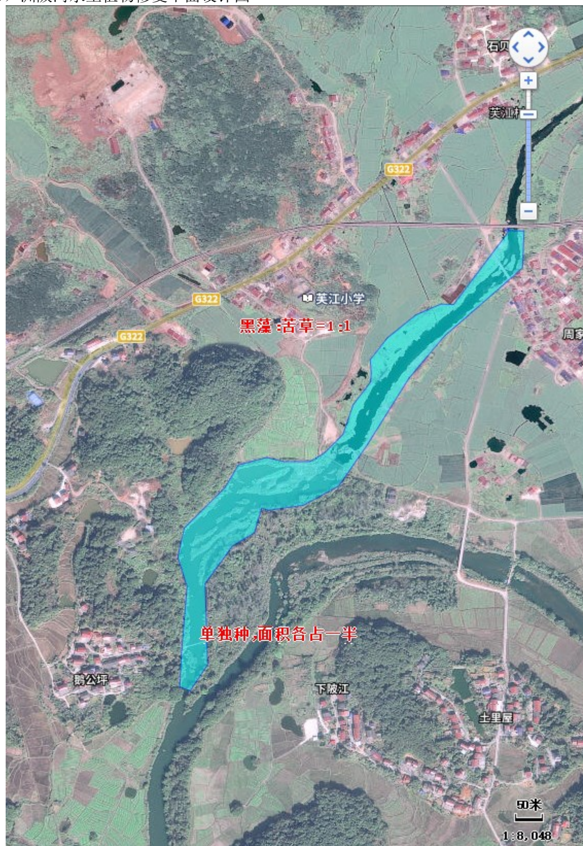
图 2-19 洲陂河水生植物修复设计图 设计平面图
