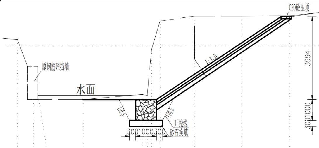
图 2-8 高陇河生态护坡断面设计 (K0+000-K0+200 一侧原本有挡墙河段)
