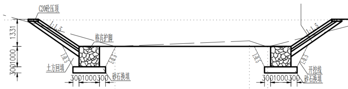
图 2-10 龙头河生态护坡断面设计
