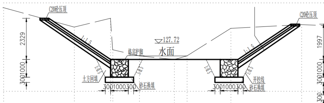
图 2-9 高陇河生态护坡断面设计 (K0+200-K0+450 河段)
