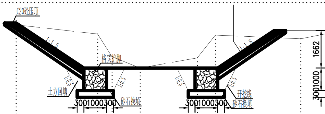
图 2-11 街里河生态护坡断面设计
