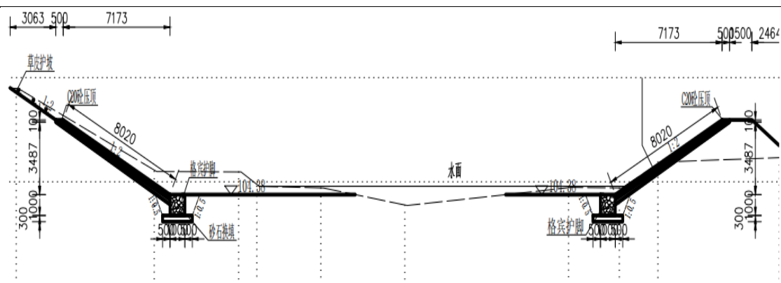
图 2-12 石联河生态护坡断面设计
