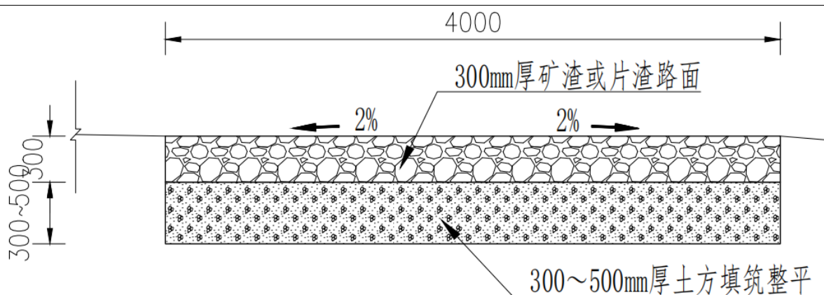
临时施工道路图 1:50
