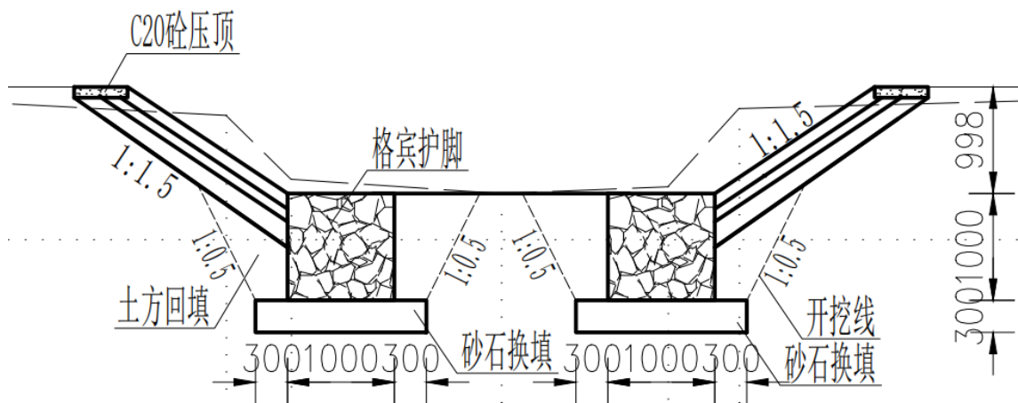
图 2-7 合湖溪生态护坡断面设计
