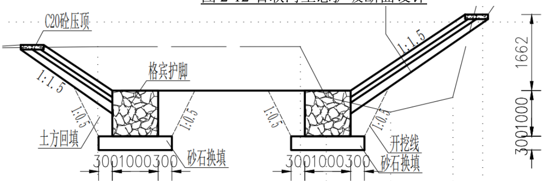
图 2-13 安坑溪生态护坡断面设计
