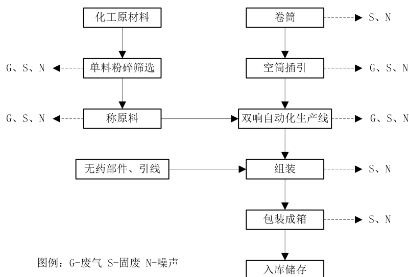
图 2-3 药物裸药效果件工艺流程及产污环节图
