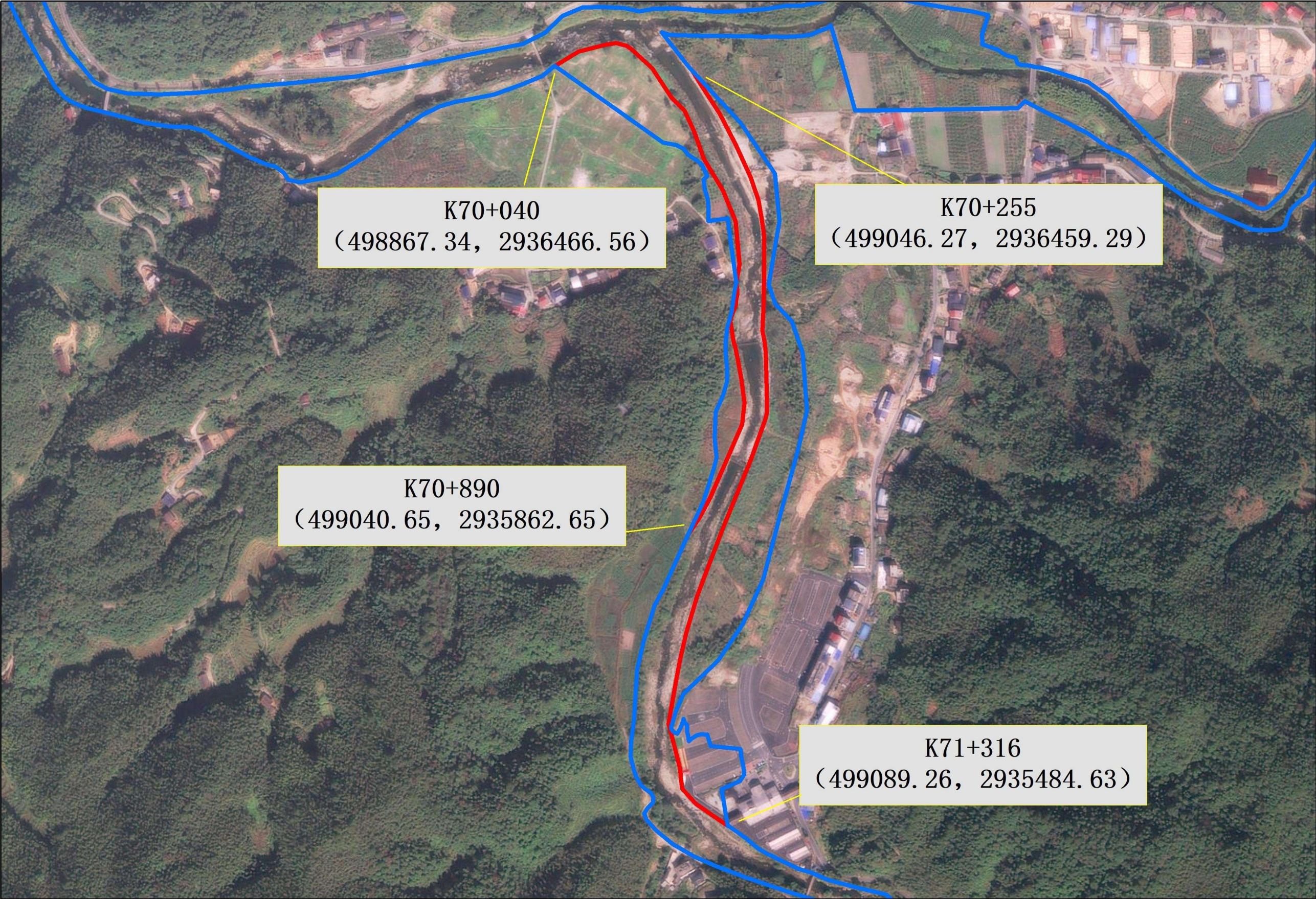
附图 4-2 (2024年底图) 沔水 (K70+040~K71+316) 河段管理范围划定成果调整前后对比图
