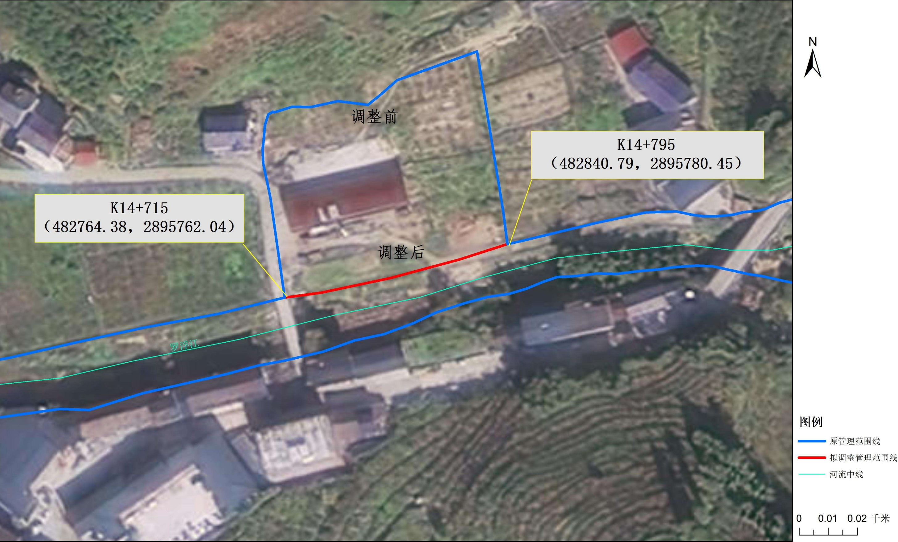
附图 4 罗浮江（K14+715-K14+795）河段管理范围划定成果调整前后对比图
