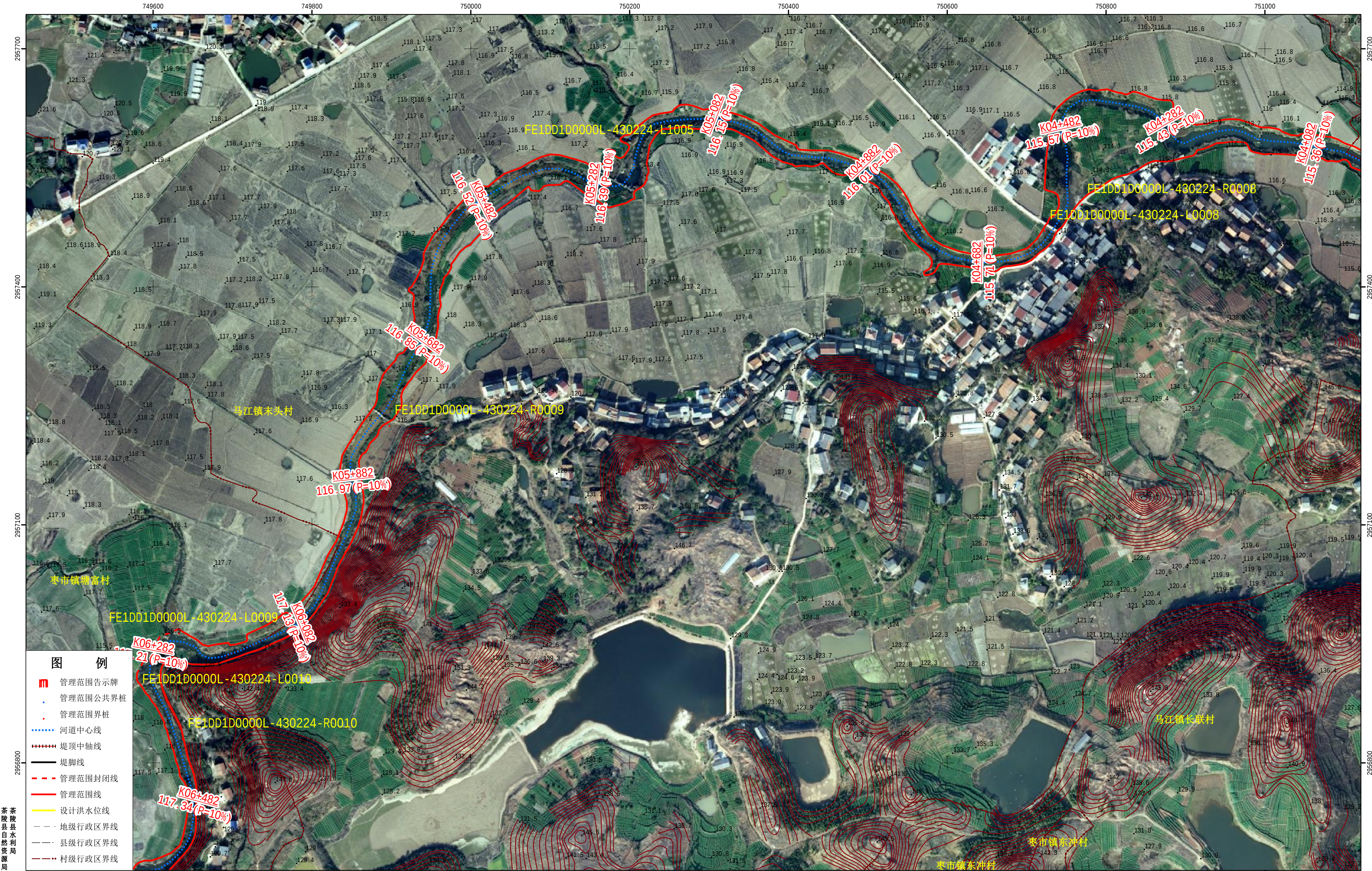
茶陵县马伏江河道管理范围划定图（三）
