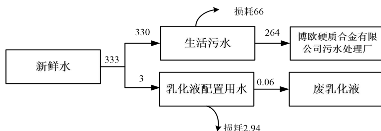
图 2-5 水平衡图（m 3 /a）
