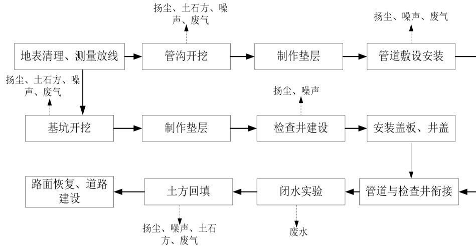
图 3.3-2 污水管网施工流程及产污环节
