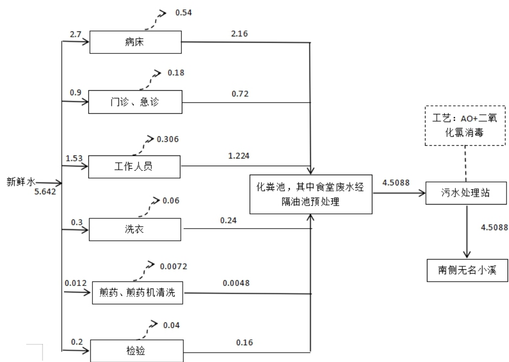
图 2-1 项目运营期水平衡图（单位 t/d）
