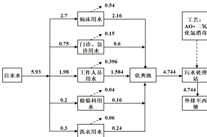
图 2-1 项目运营期水平衡图 (单位 t/d)
