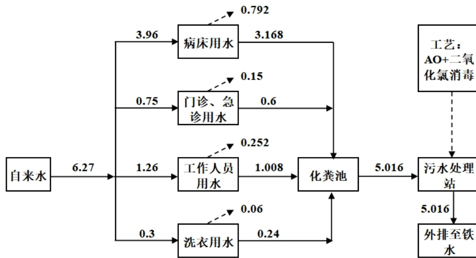
图 2-1 项目运营期水平衡图（单位 t/d）
