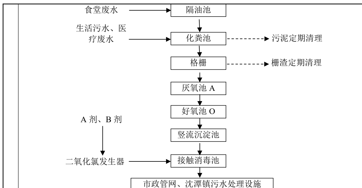
图 4-1 项目污水处理系统工艺流程图
