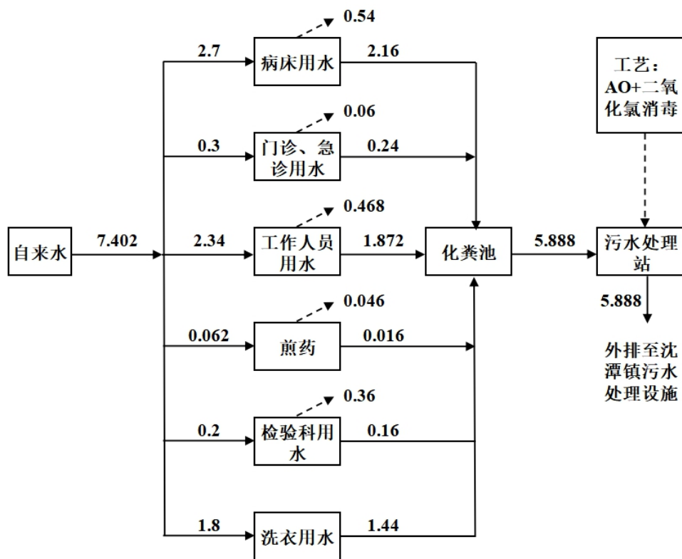
图 2-1 项目运营期水平衡图（单位 t/d）
