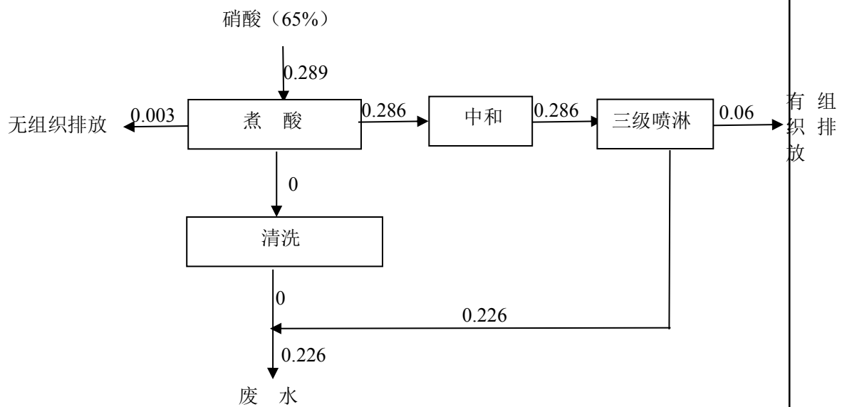
图 2-4 C 硝酸（以 N 计）平衡示意图 单位：t/a
