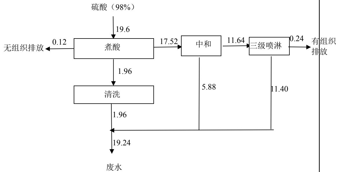
图 2-4 B 硫酸平衡示意图 单位：t/a
