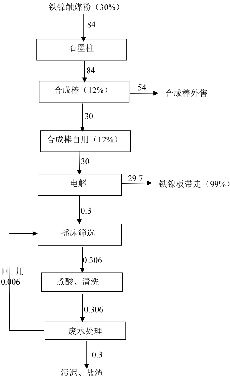
图 2-5 镍元素平衡示意图 单位：t/a
