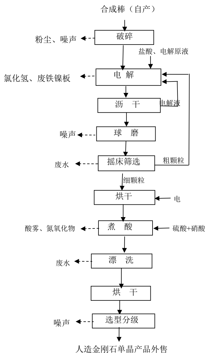
图 2-3 人造金刚石单晶生产工艺流程及产污节点示意图
