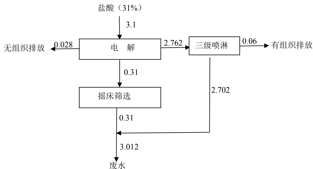
图 2-4 A 氯化氢 (不含污水处理用酸) 平衡示意图
