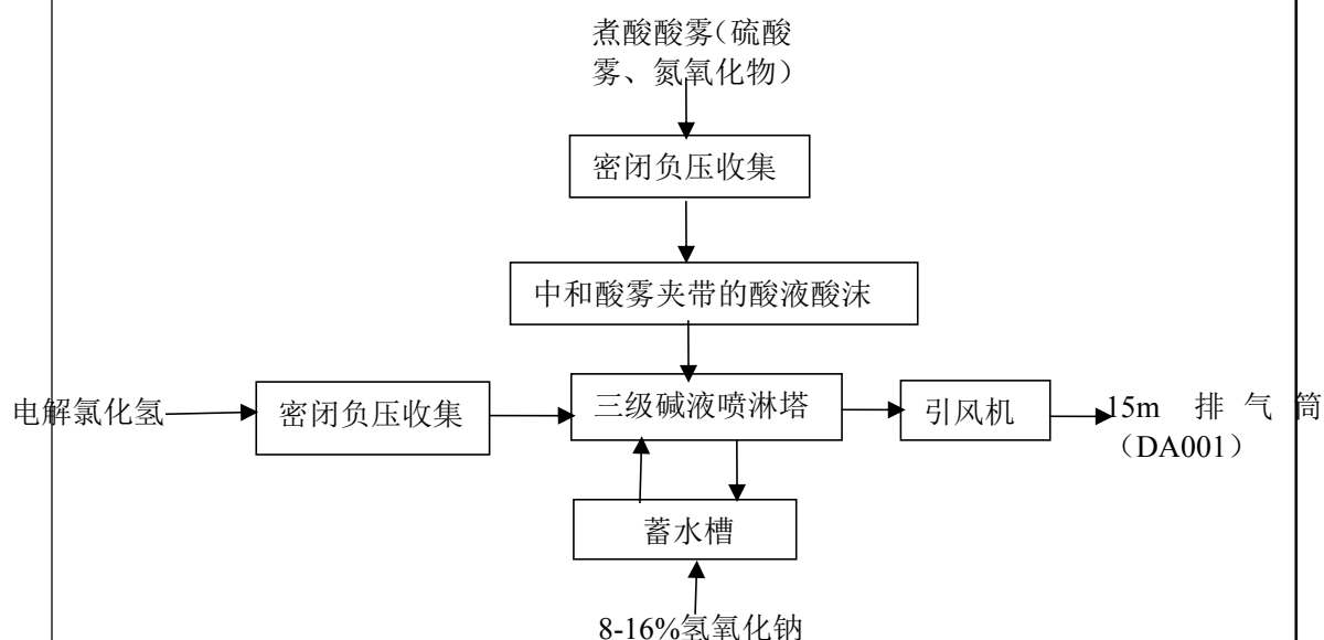
图 4-1 电解、煮酸酸雾净化工艺流程示意图
