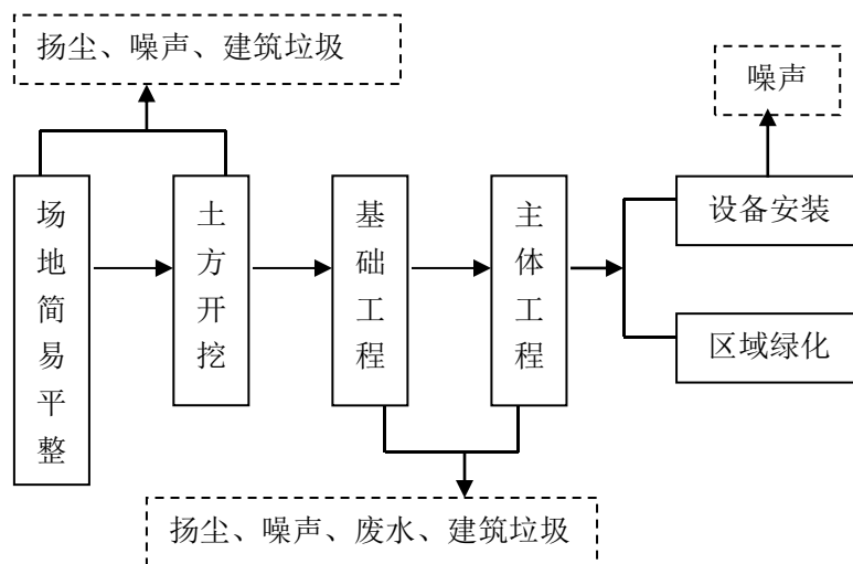
图 2-1 施工流程及产污节点示意图
