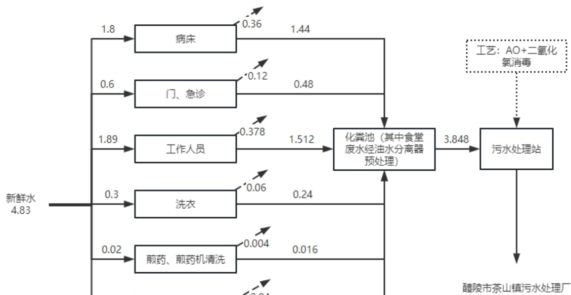
图 2-1 项目运营期水平衡图（单位 t/d）
