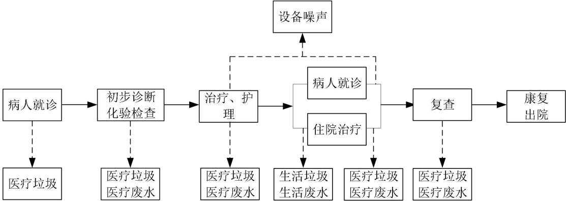
图 2-1 医院工艺流程及产污环节图
