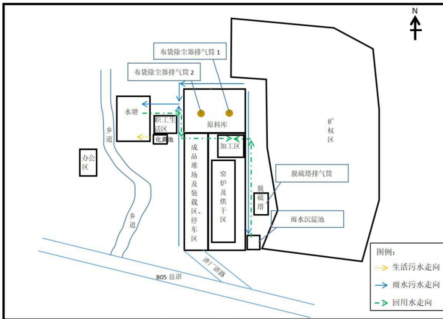
附图 2 项目厂区平面布置示意图
