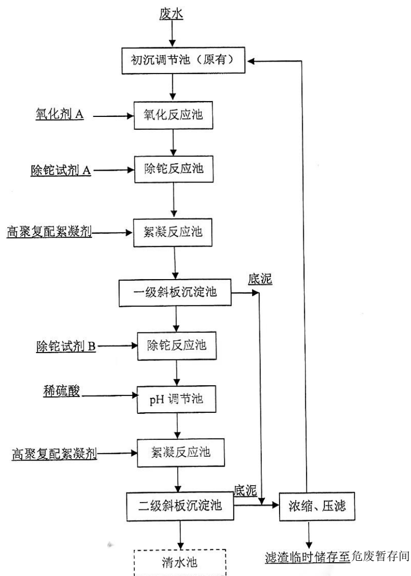
图 4-2 除铊设施工艺流程图
