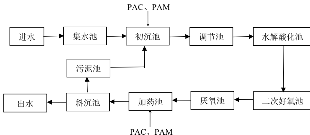
图 3-3 废水处理站工艺流程
