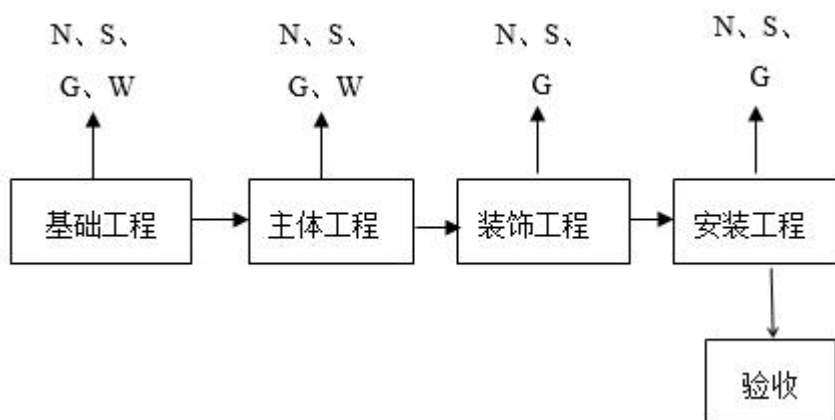
图 4-5 施工期工艺流程及产污节点图
