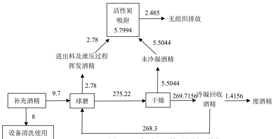
图 4-4 本项目酒精平衡图（单位：t/a）
