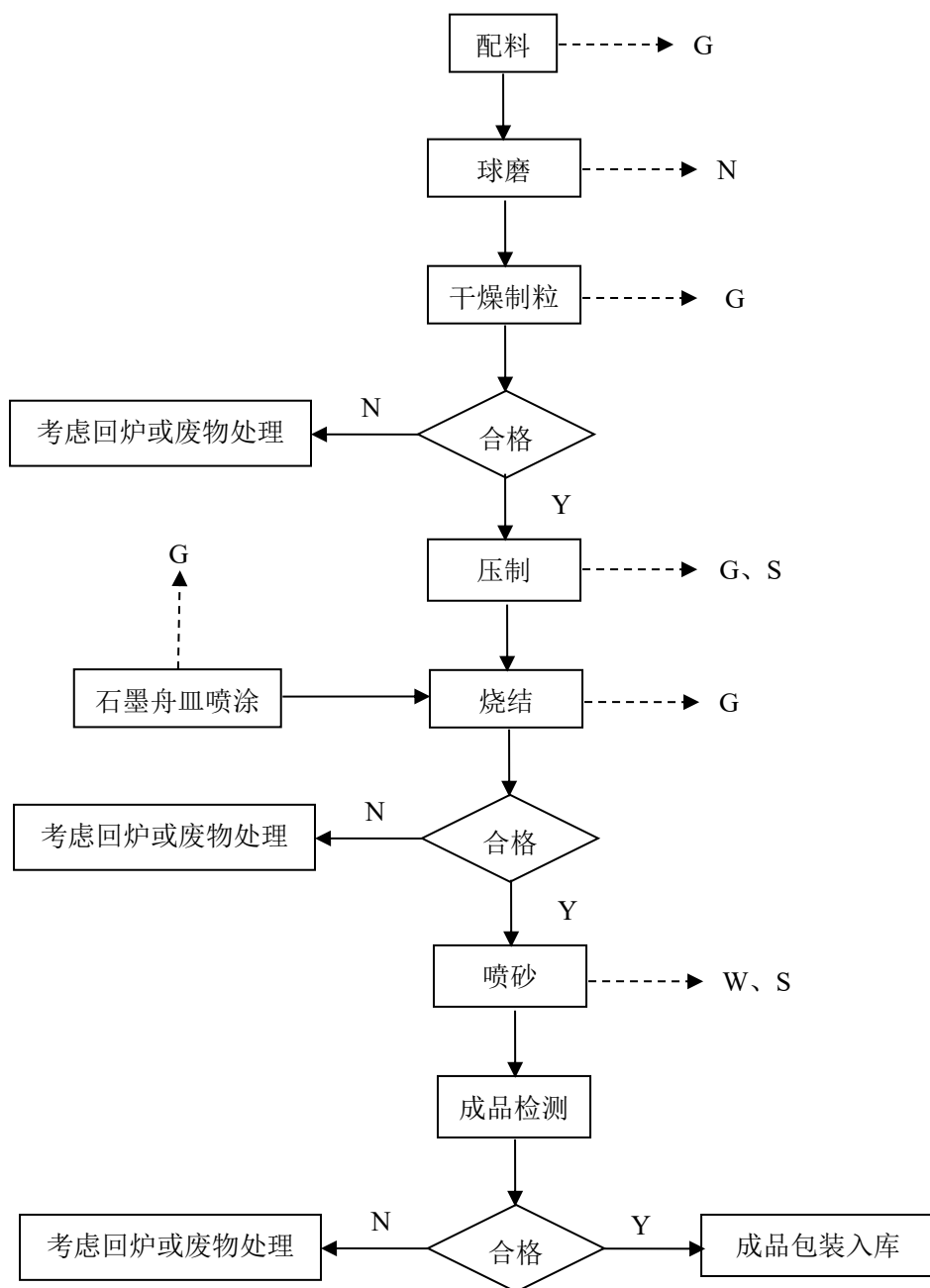
图 3-1 硬质合金工程材料工艺流程以及产污节点图
