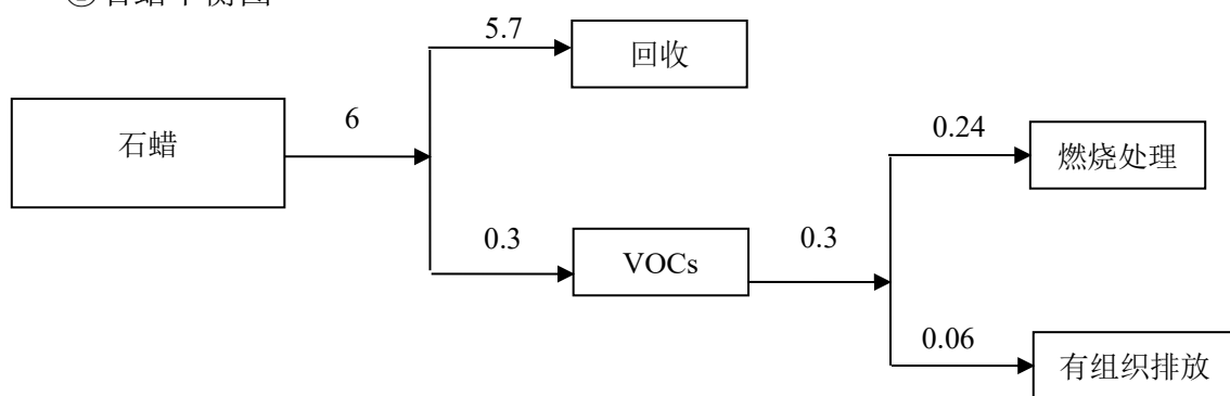
图 4-2 本项目成型剂（石蜡）平衡图（单位：t/a）
