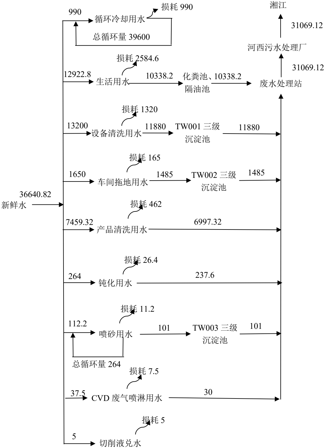
图 4-1 本项目改扩建后全厂水平衡图 (单位: t/a)
