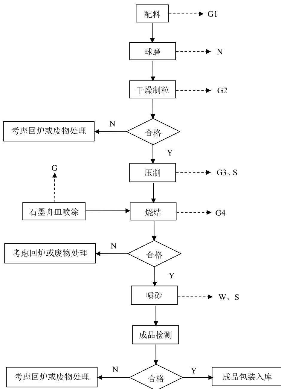
图 4-6 硬质合金工程材料工艺流程以及产污节点图
