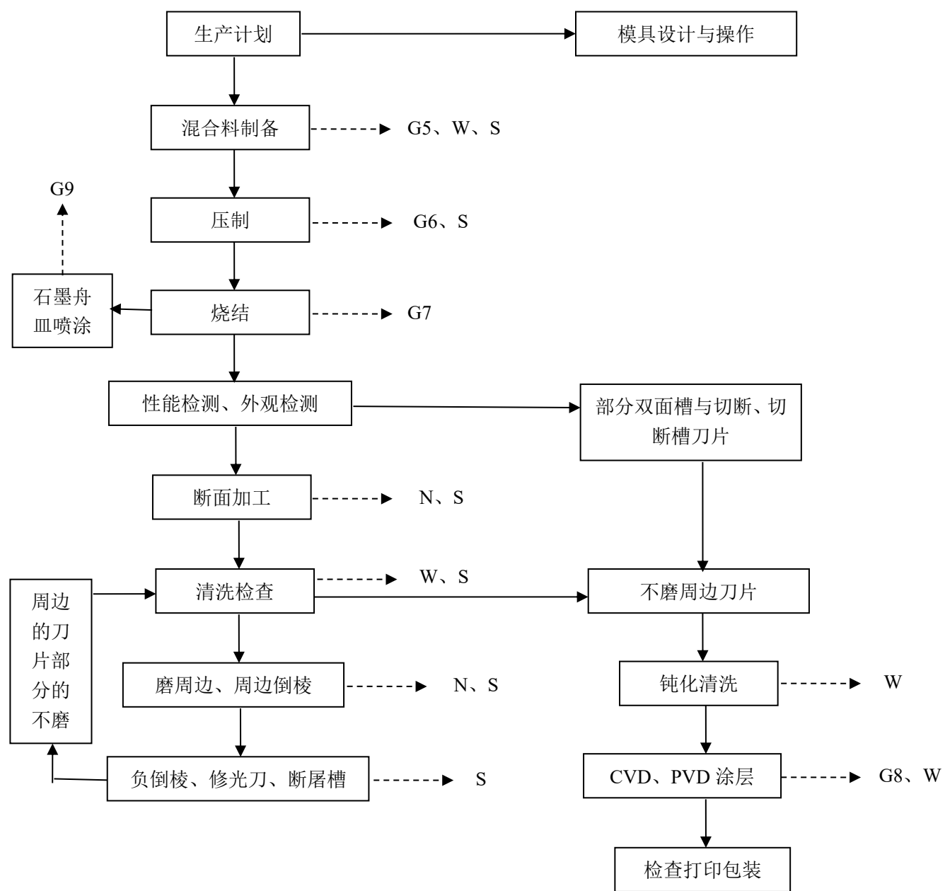
图 4-7 数控刀片工艺流程以及产污节点图
