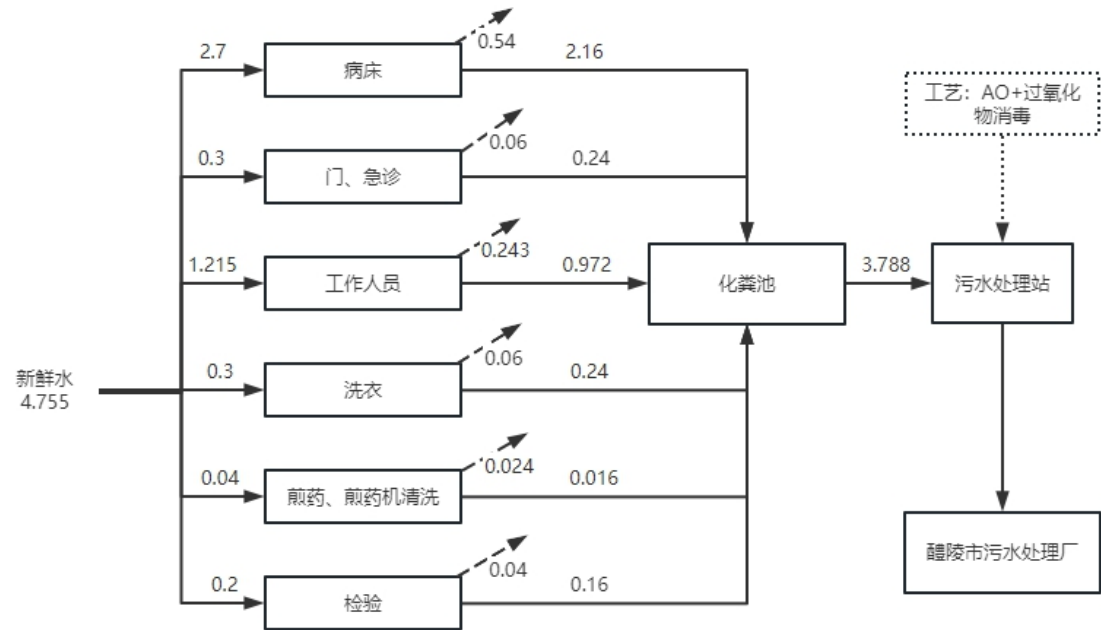
项目水平衡图如下：
