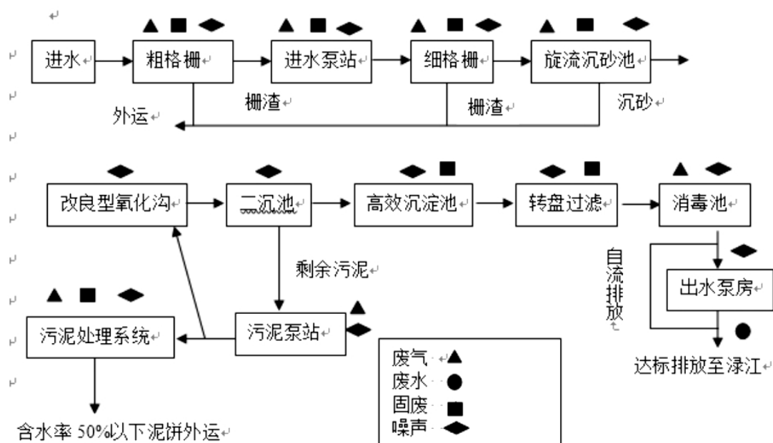
图 4-2 醴陵市污水处理厂工艺流程图
