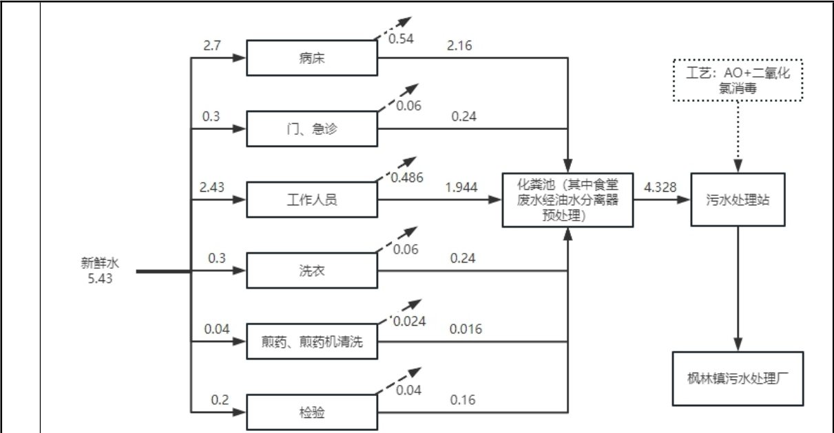
图 2-1 项目运营期水平衡图 (单位 t/d)
