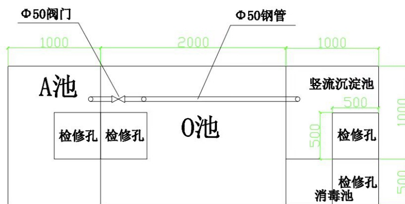
顶板平面图 4米*1.5米*2米钢箱
