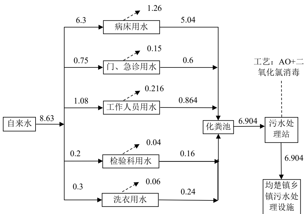
图 2-1 项目运营期水平衡图（单位 t/d）
