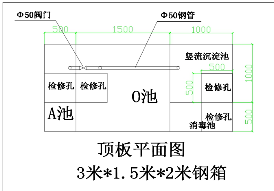
图 4-2 项目污水处理站平面布置图
