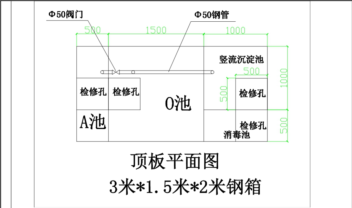
图 4-2 项目污水处理站平面布置图
