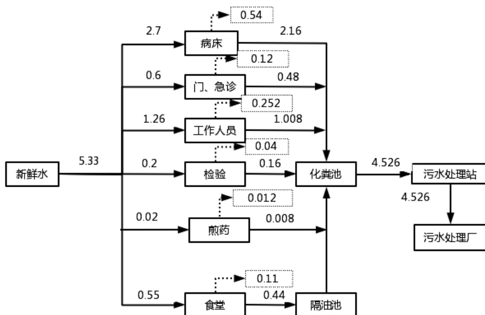
图 2-1 项目运营期水平衡图（单位 t/d）
