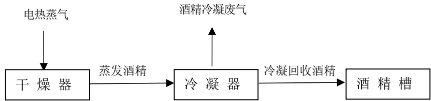
图 6-1 酒精冷凝回收工艺流程图
