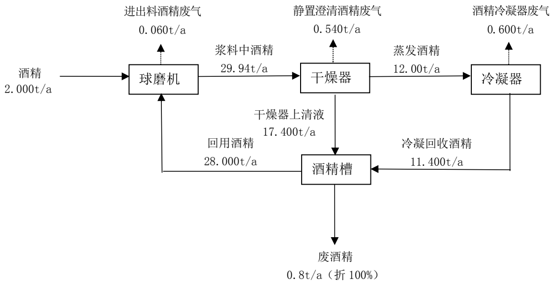
图 3-2 项目酒精平衡图
