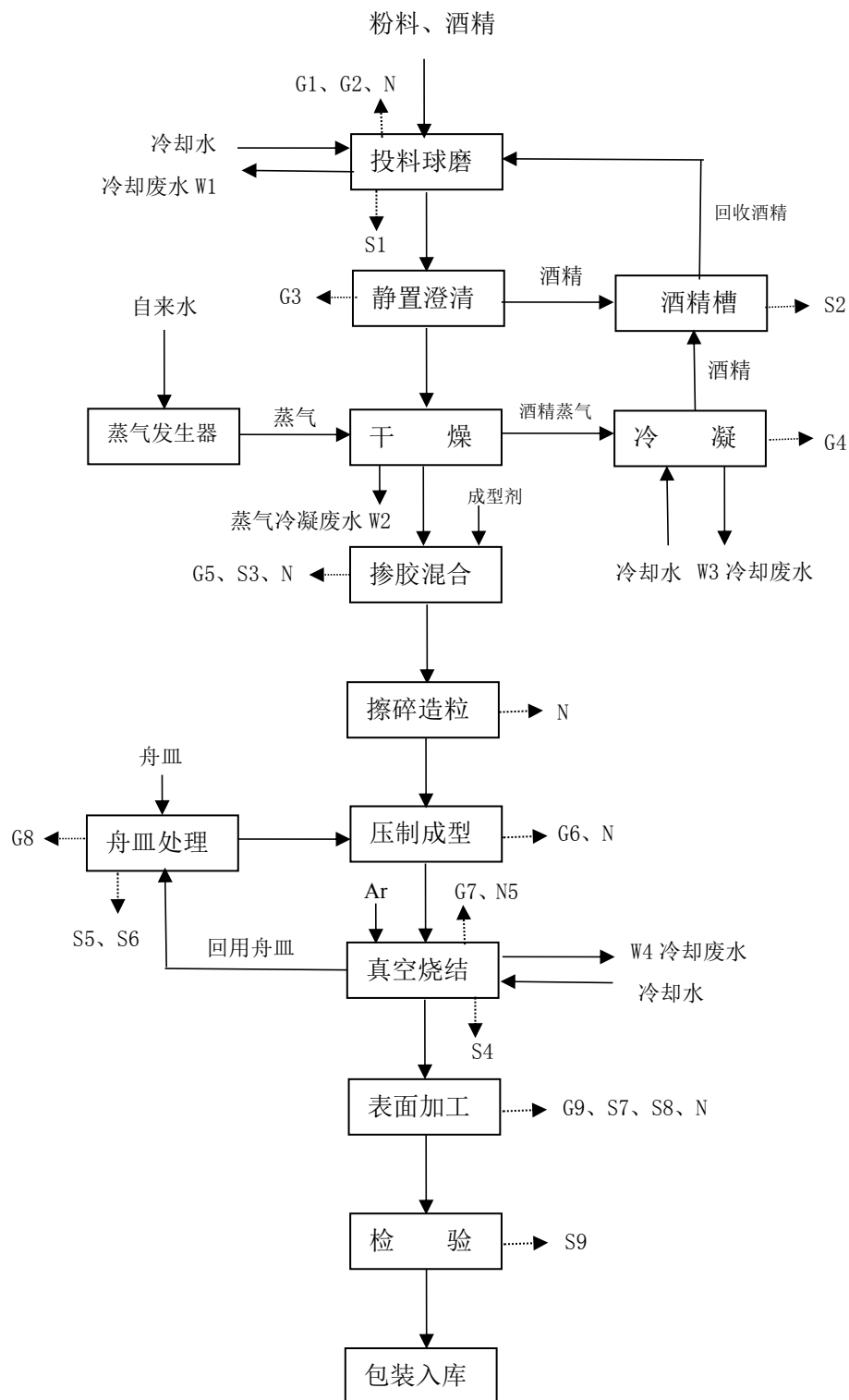
图3-1 生产工艺流程及产排污节点图
