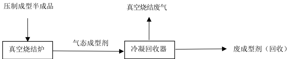
图 6-2 成型剂冷凝回收工艺流程图
