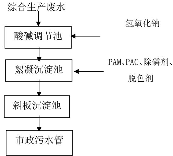
图 6.1-3 项目综合生产水处理工艺流程
