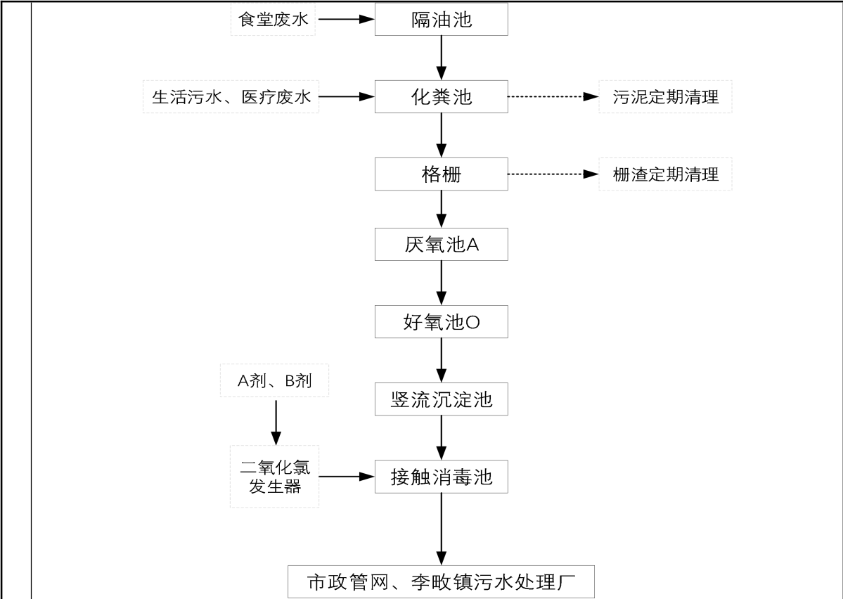
图 4-1 项目污水处理系统工艺流程图
