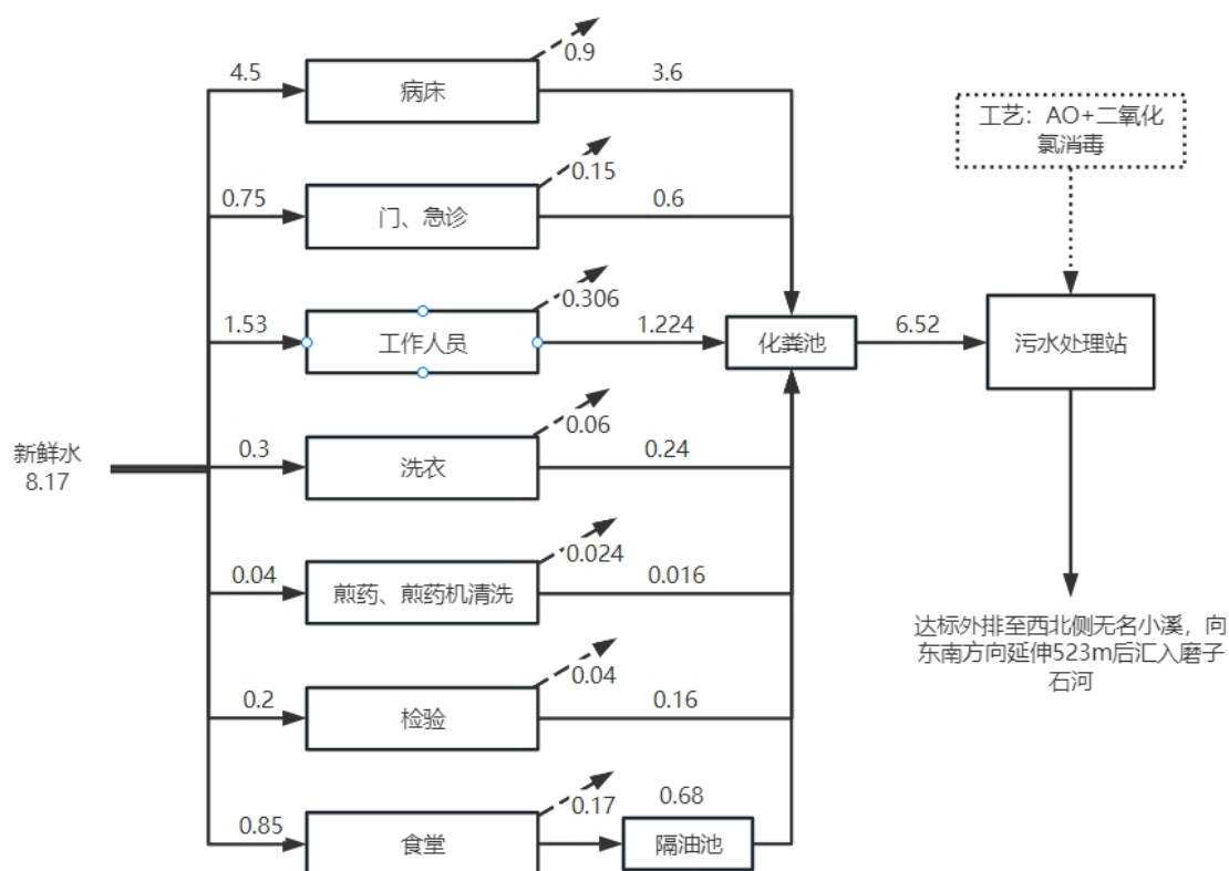
图 2-1 项目运营期水平衡图（单位 t/d）
