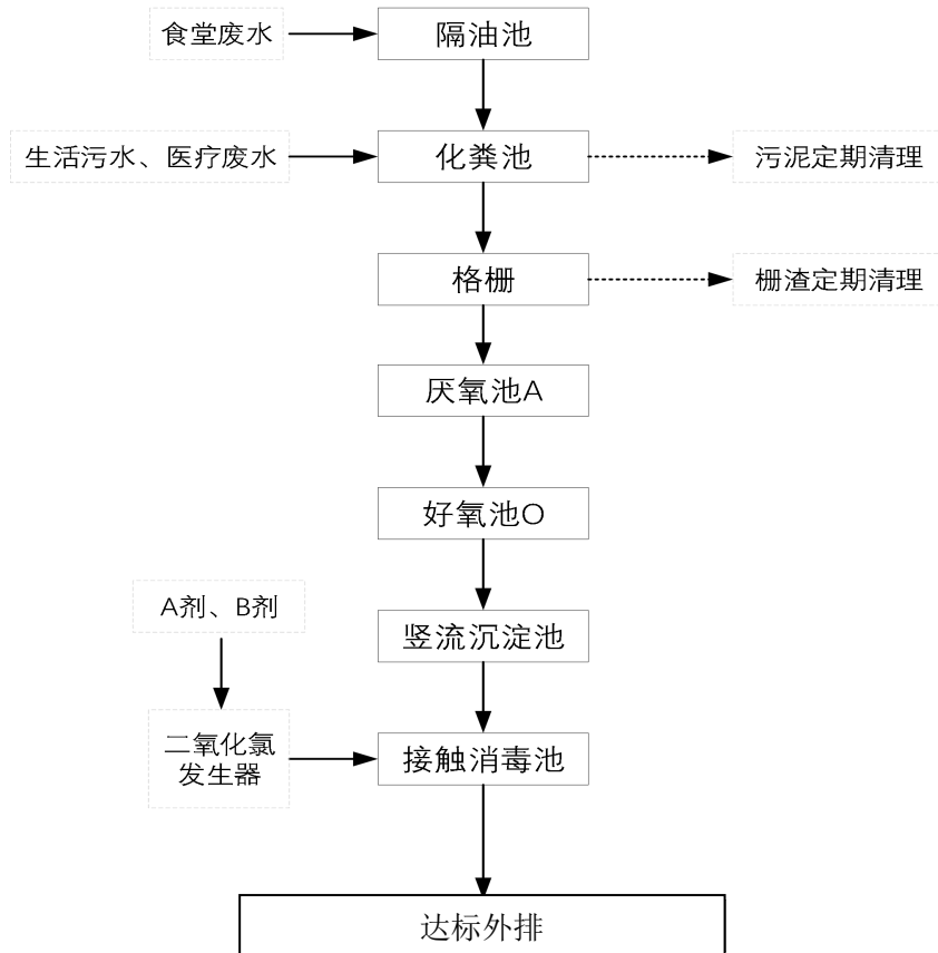
图 4-1 项目污水处理系统工艺流程图
