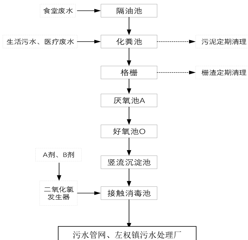
图 4-1 项目污水处理系统工艺流程图
