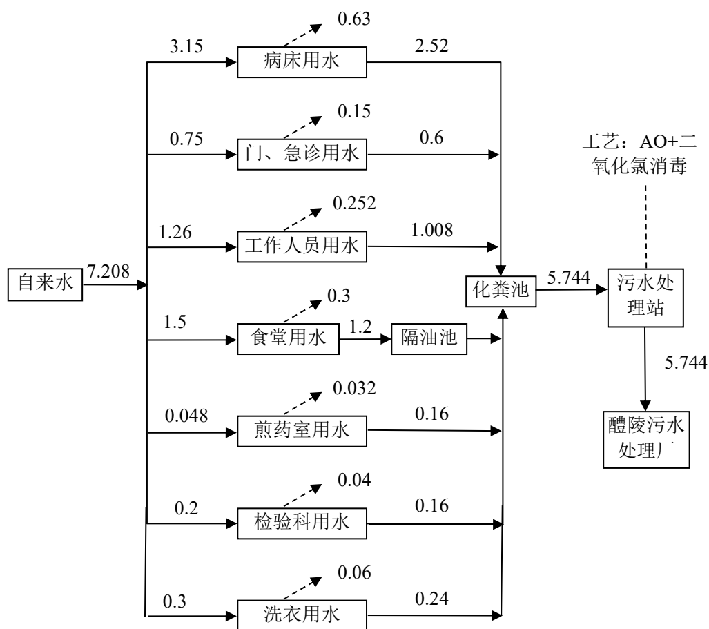
图 2-1 项目运营期水平衡图（单位 t/d）
