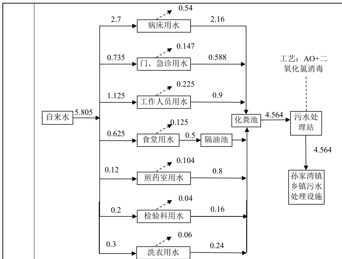
图 2-1 项目运营期水平衡图（单位 t/d）
