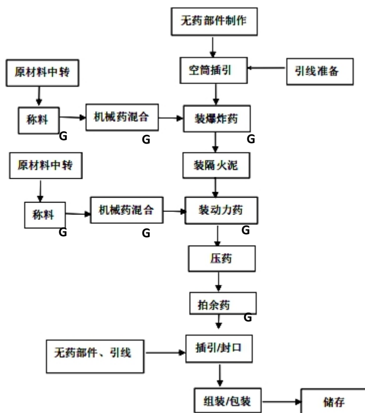
图 2-4 升空类（火箭）生产工艺流程及产污环节图
