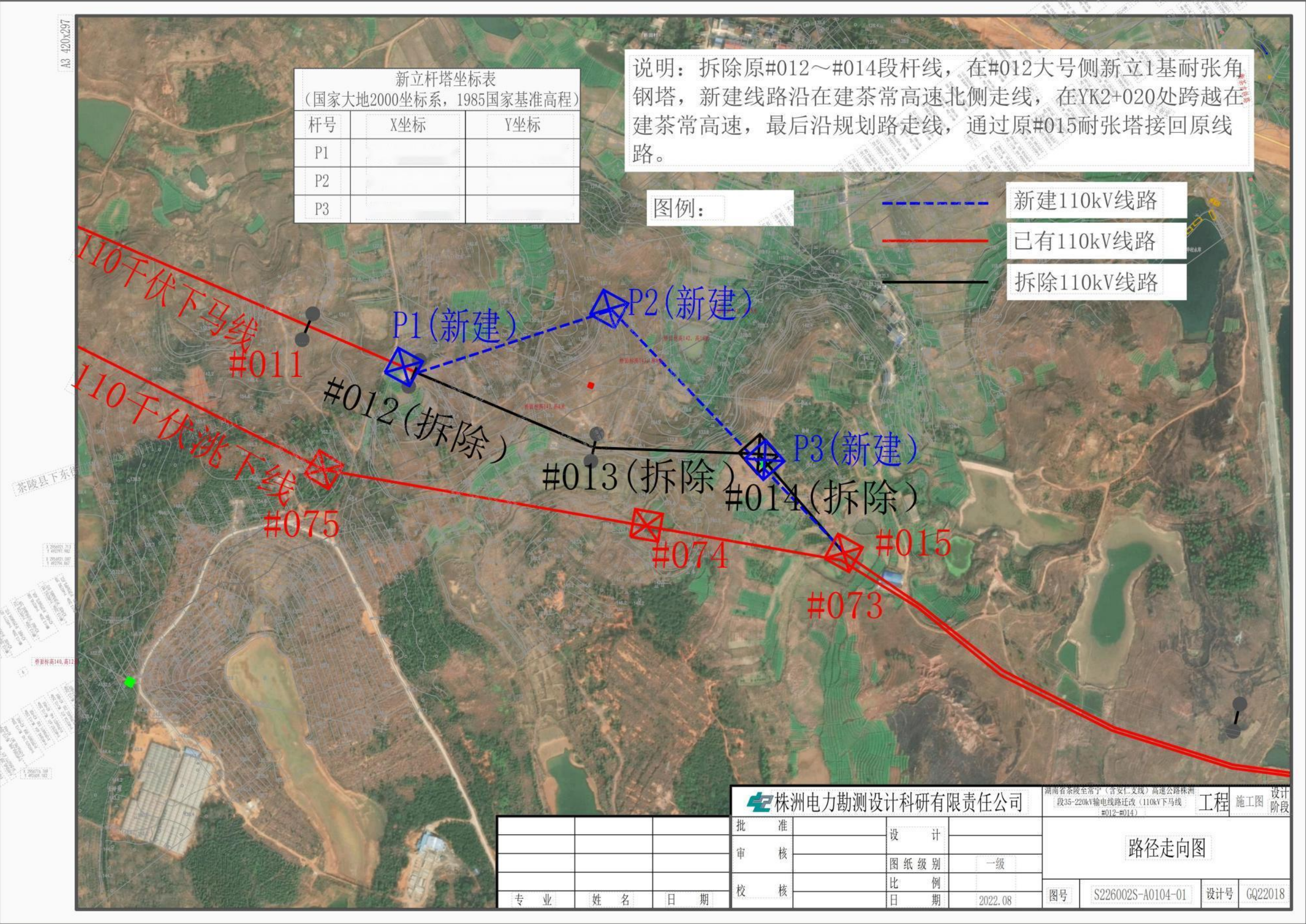
附图 2 线路路径方案图
