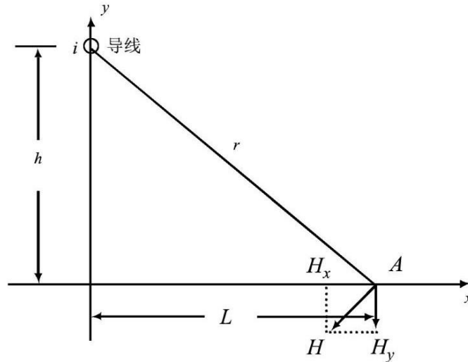
图 4 磁场向量图
