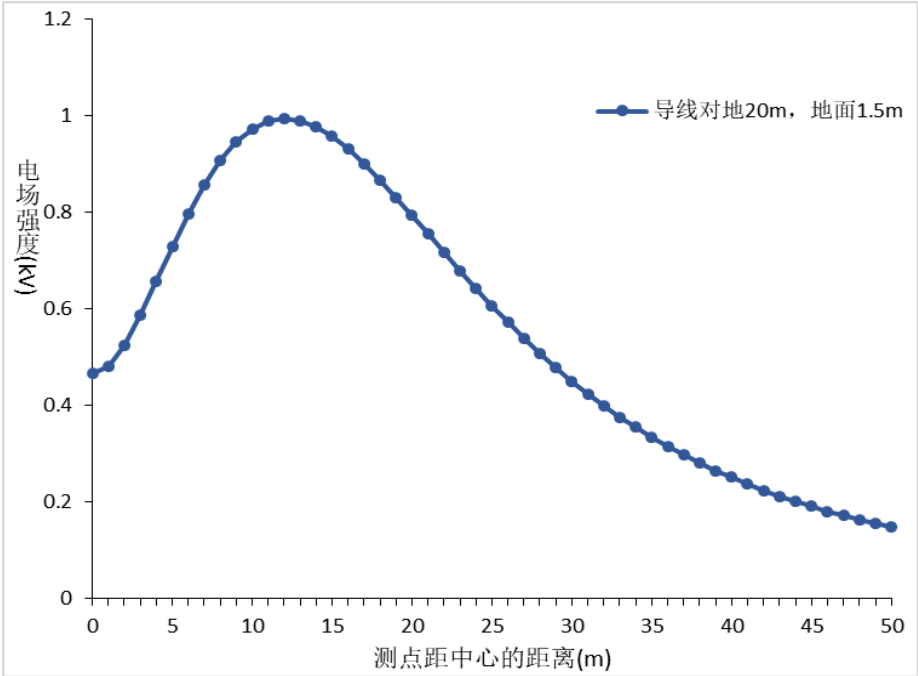
图 5 本工程线路工频电场强度预测结果
