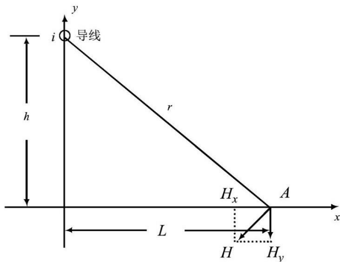
图 3 磁场向量图
