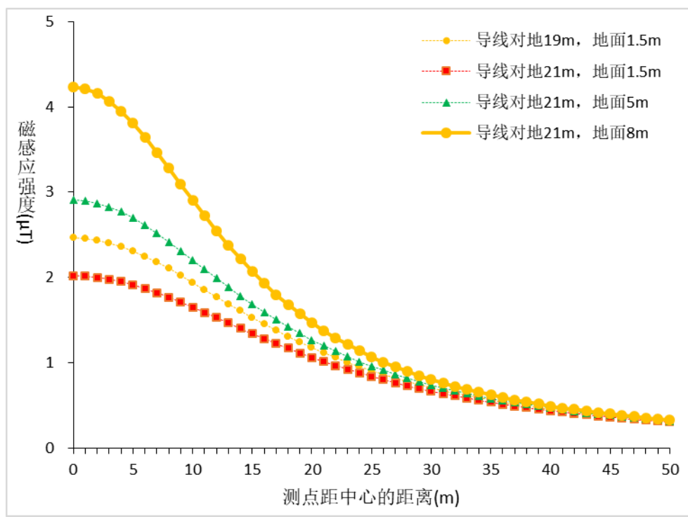
图 6 本工程线路工频磁感应强度预测结果
