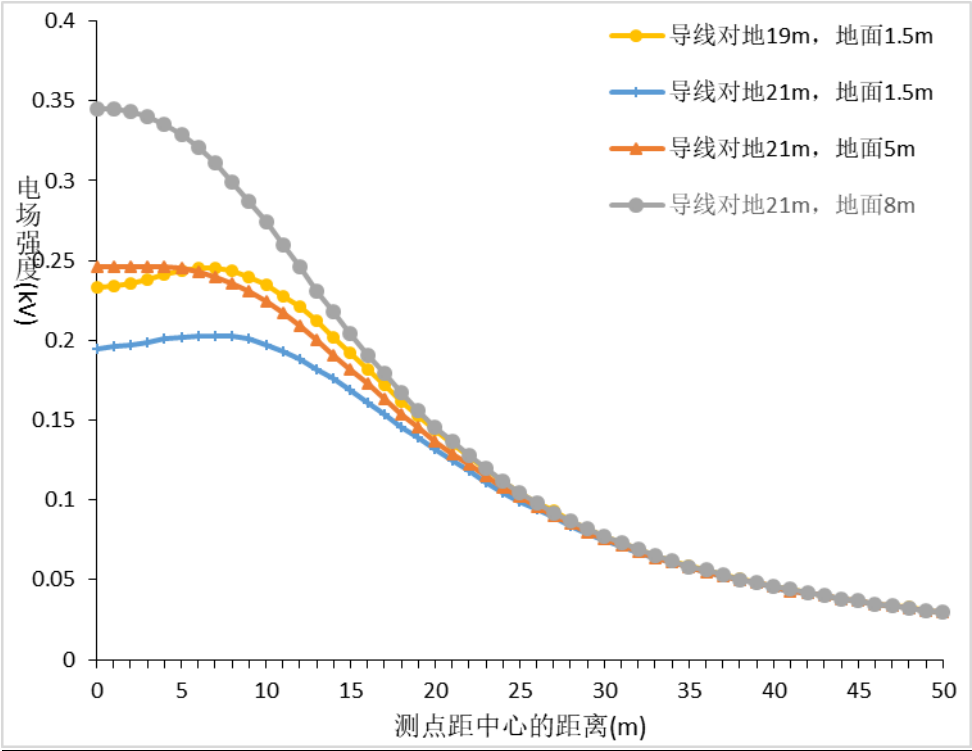
图 5 本工程线路工频电场强度预测结果
