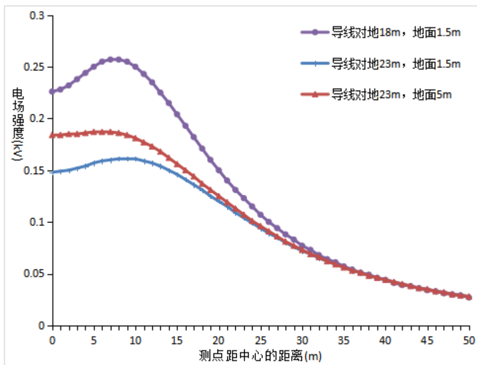
图 5 本工程线路工频电场强度预测结果
