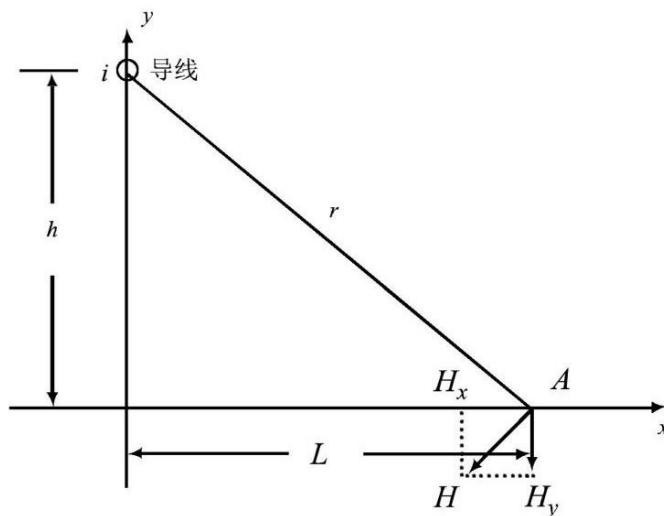
图 3 磁场向量图
