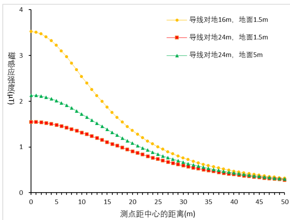
图 6 本工程 110kV 单回线路工频磁感应强度预测结果
