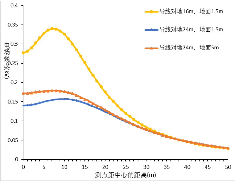
图 5 本工程 110kV 单回线路工频电场强度预测结果
