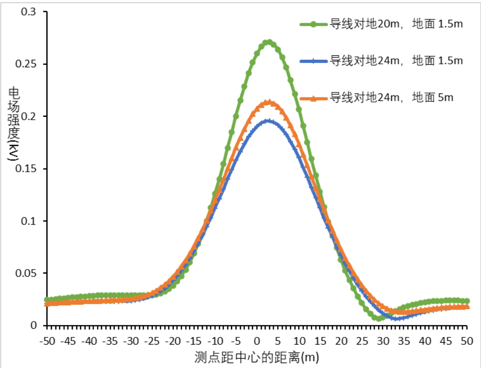
图7 本工程 110kV 双回线路（右侧送电）工频电场强度预测结果
