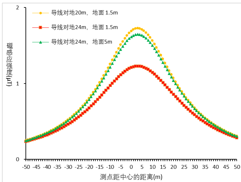
图8 本工程110kV双回线路（右侧送电）工频磁感应强度预测结果
