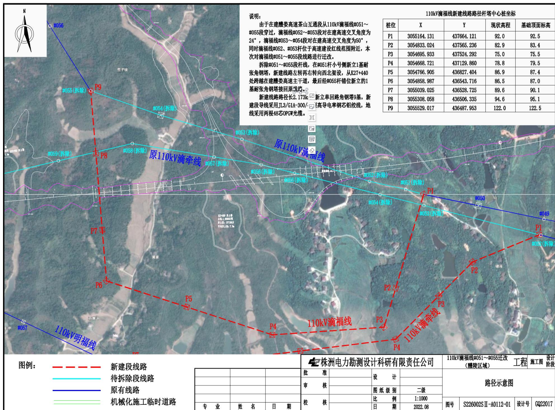
附图 2 线路路径方案图
