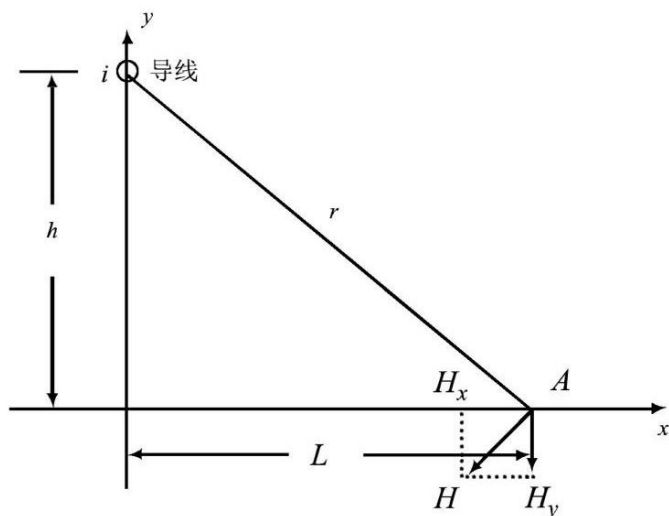
图 4 磁场向量图
