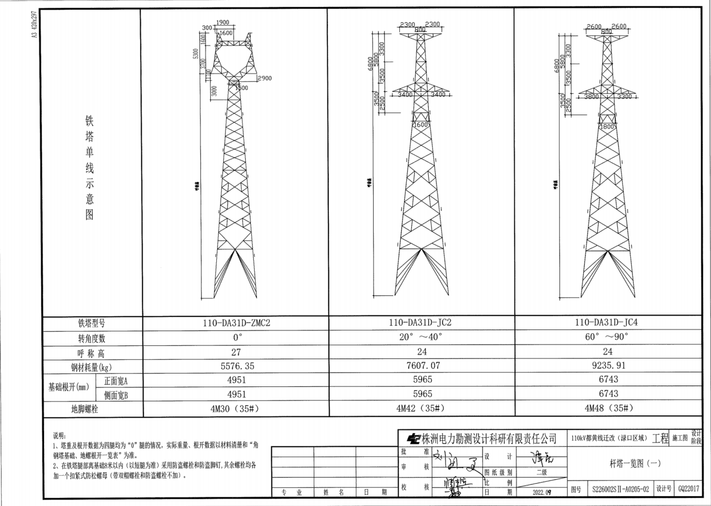
附图 4 杆塔图
