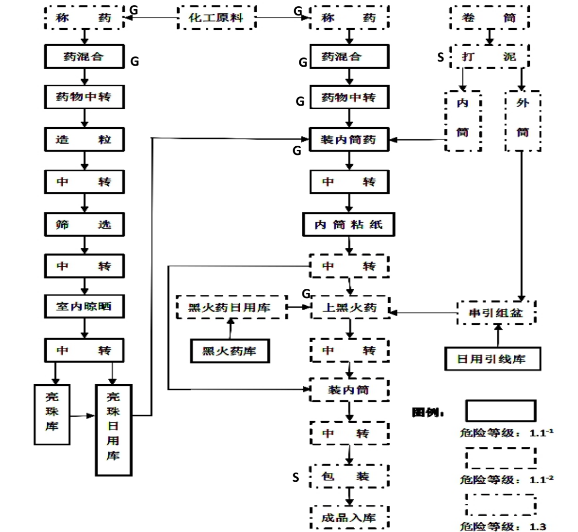
图 2-3 组合类烟花生产工艺流程及产污环节图
