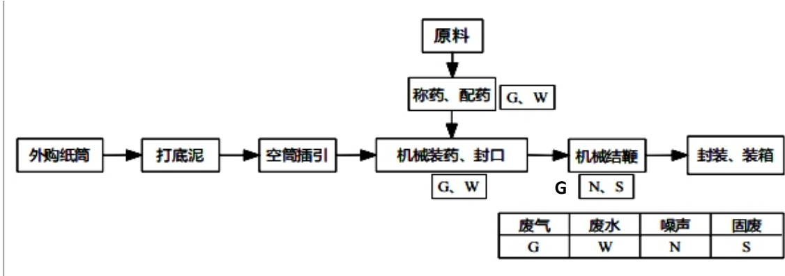
图 2-2 鞭炮生产工艺流程及产污环节图
