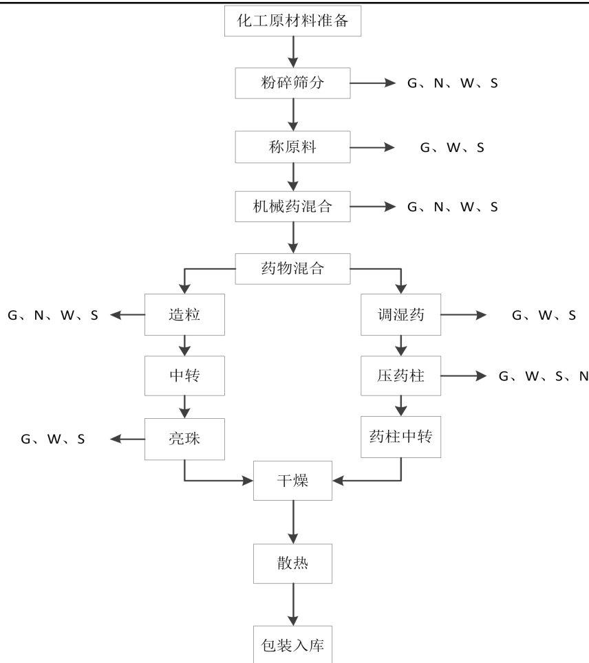
图 2-4 亮珠工艺流程图及产污节点图
